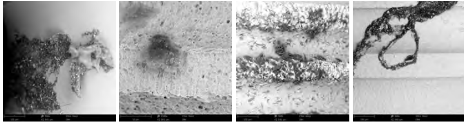
Organische Verunreinigungen auf steril verpackten Implantaten - REM Bilder © 2016-2019 CleanImplant Foundation | Dr. Dirk U. Duddeck | mmri.berlin
